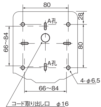
取付面寸法図
